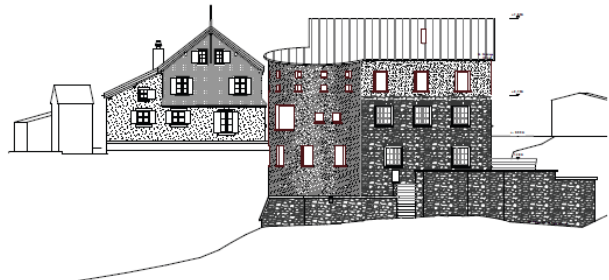
Ansicht Südwest 1:100
