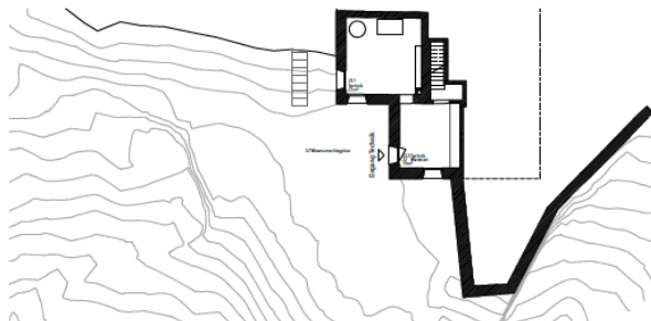
2. Untergeschoss 1:100
