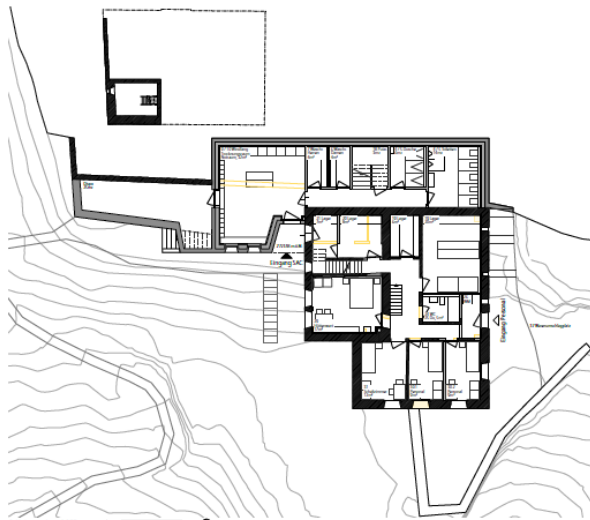
1. Untergeschoss 1:100
