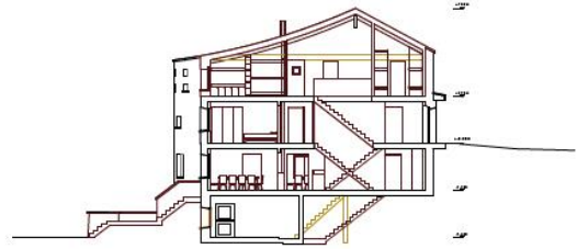
Schnitt A-A 1:100
