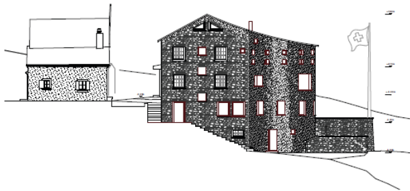
Ansicht Nordwest 1:100
